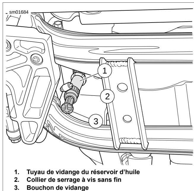
Figure 1-4. Tuyau de vidange du réservoir d'huile
