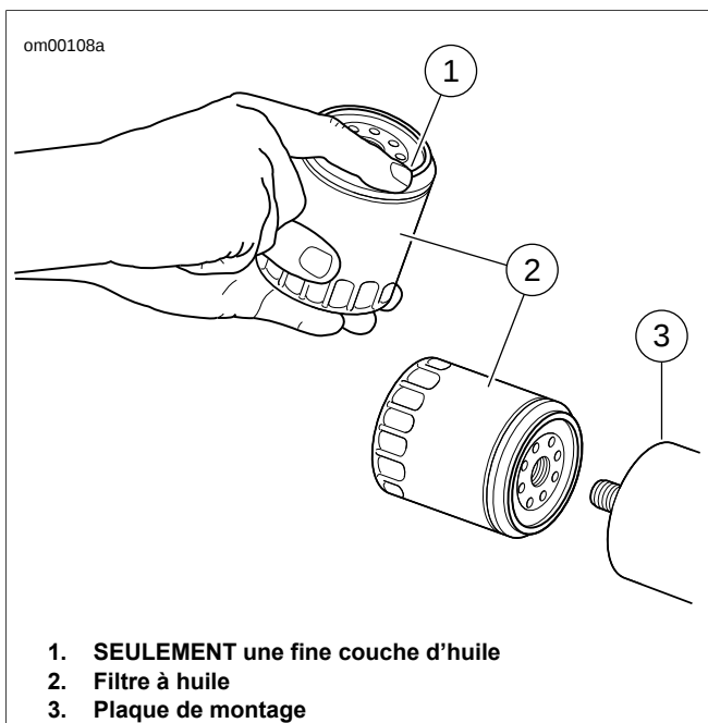
Figure 1-7. Application d'une couche mince d'huile
