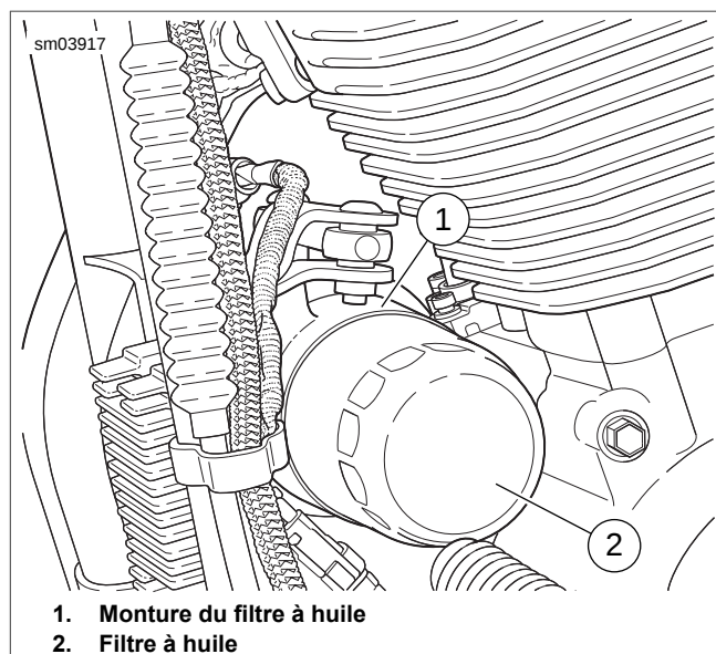
Figure 1-6. Filtre à huile
