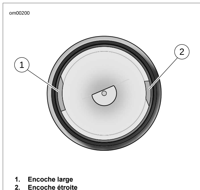
Figure 1-2. Encoches du bouchon de remplissage
